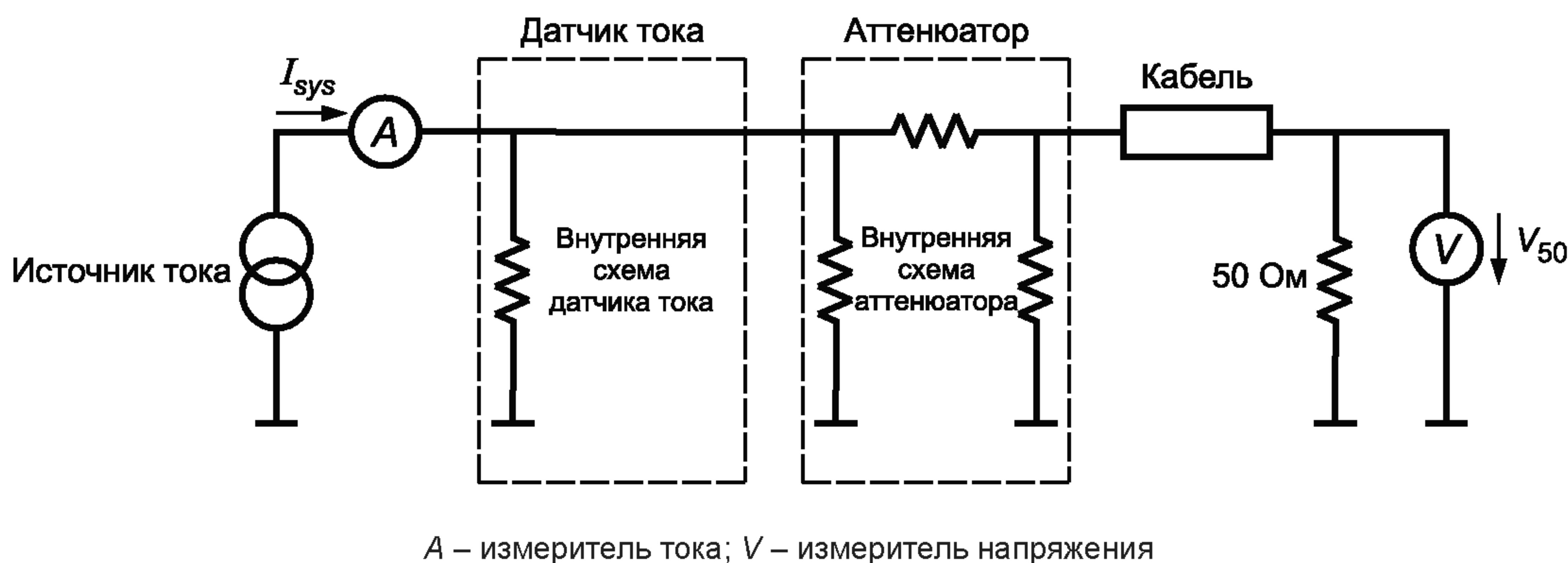
Рисунок В.4 – Схема определения низкочастотного передаточного сопротивление системы измерения тока
