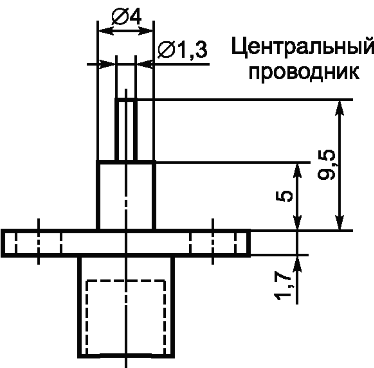
Соединитель. Приблизительно 2:1
