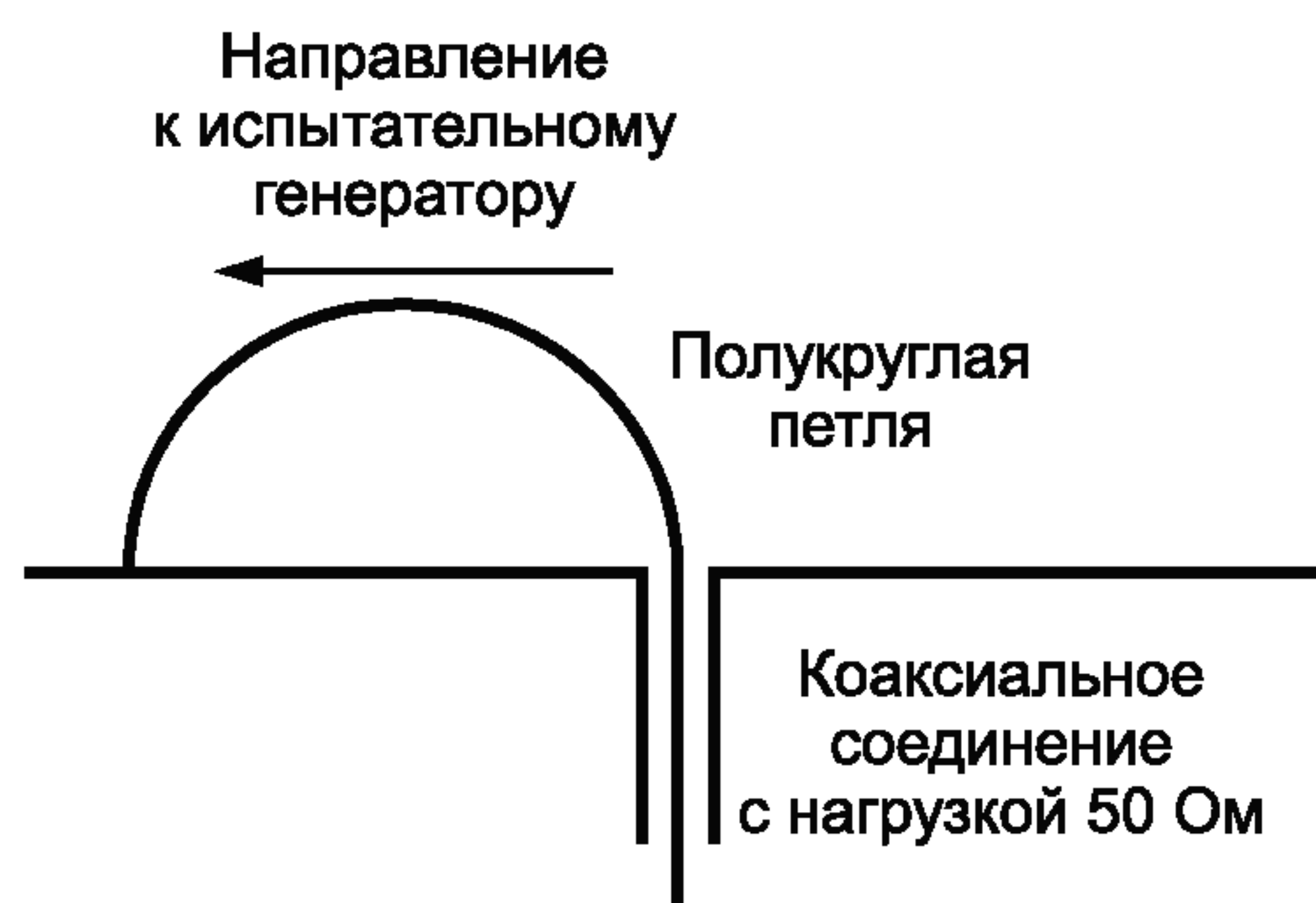
Рисунок D.3 – Полукруглая петля на пластине заземления
