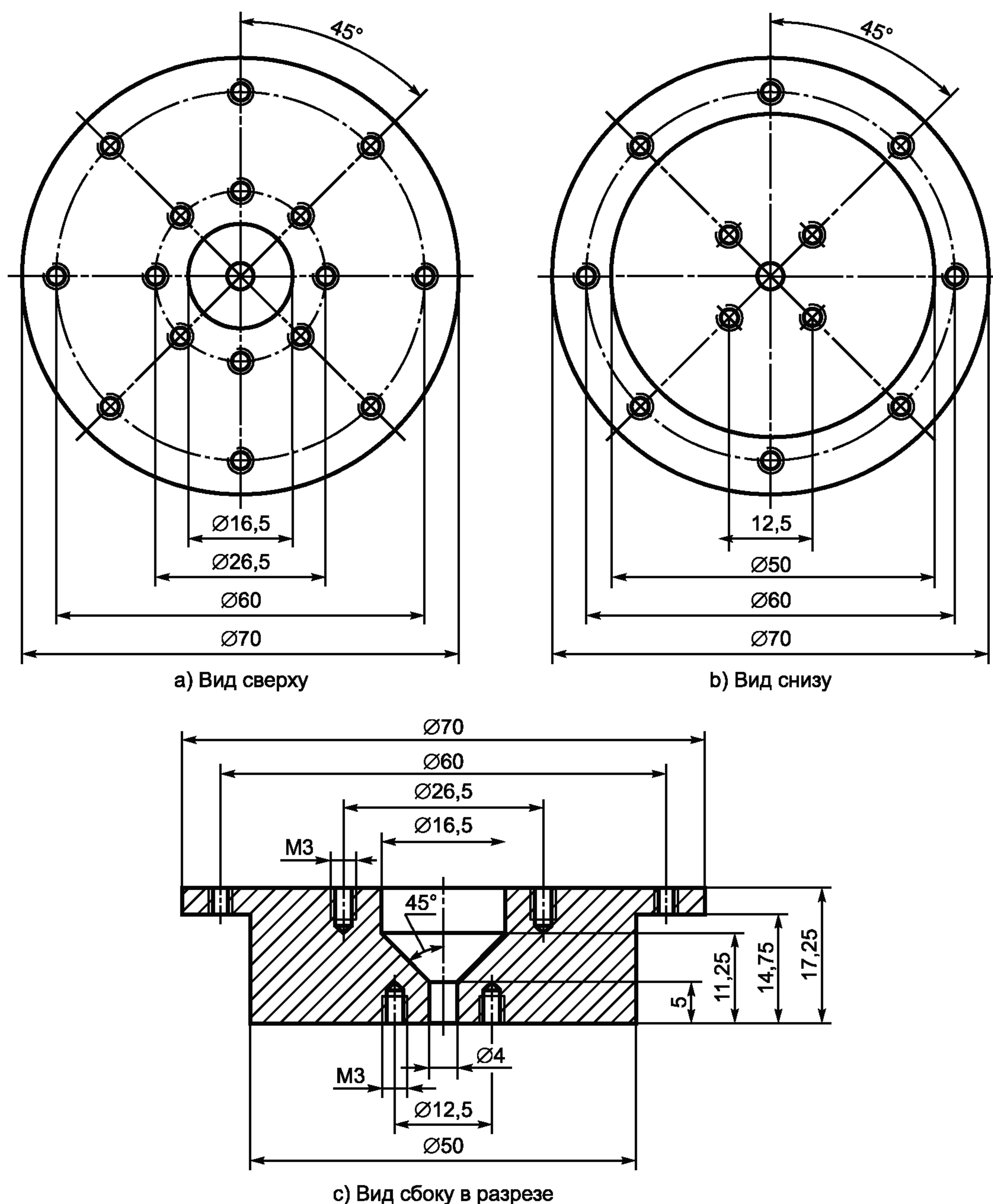
Рисунок С.1 – Чертеж коаксиального датчика (лист 1 из 5)
